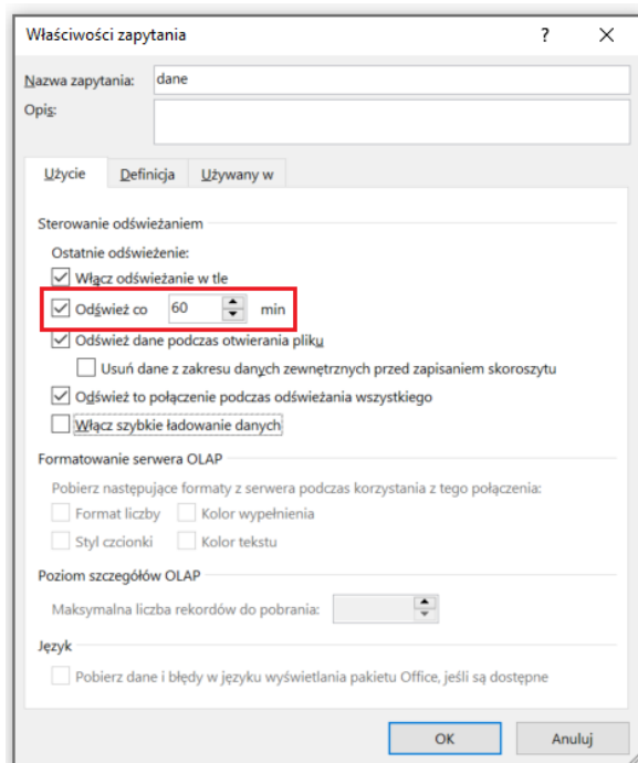
Rysunek ODD. 14 Odświeżanie tabeli co określony czas
